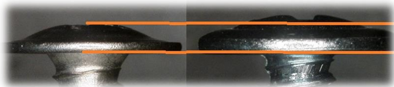
SL-DRIVE 高さ 1.5mm シンワッシャードリル 高さ 2.3mm
